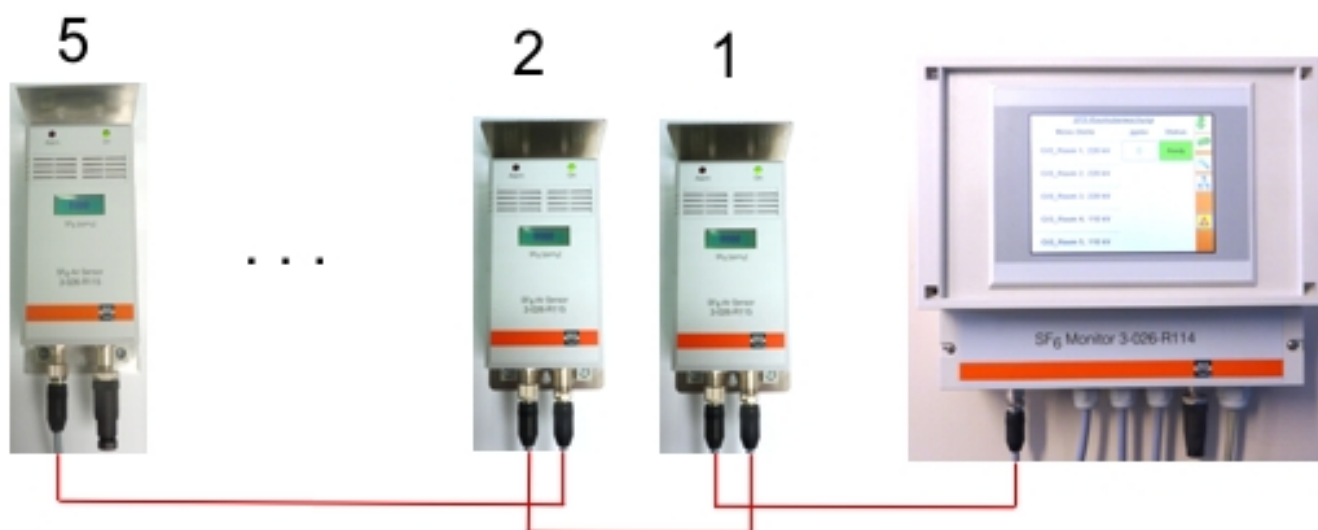
Рисунок 2.1 Пример подключения (Подключение к сети).
